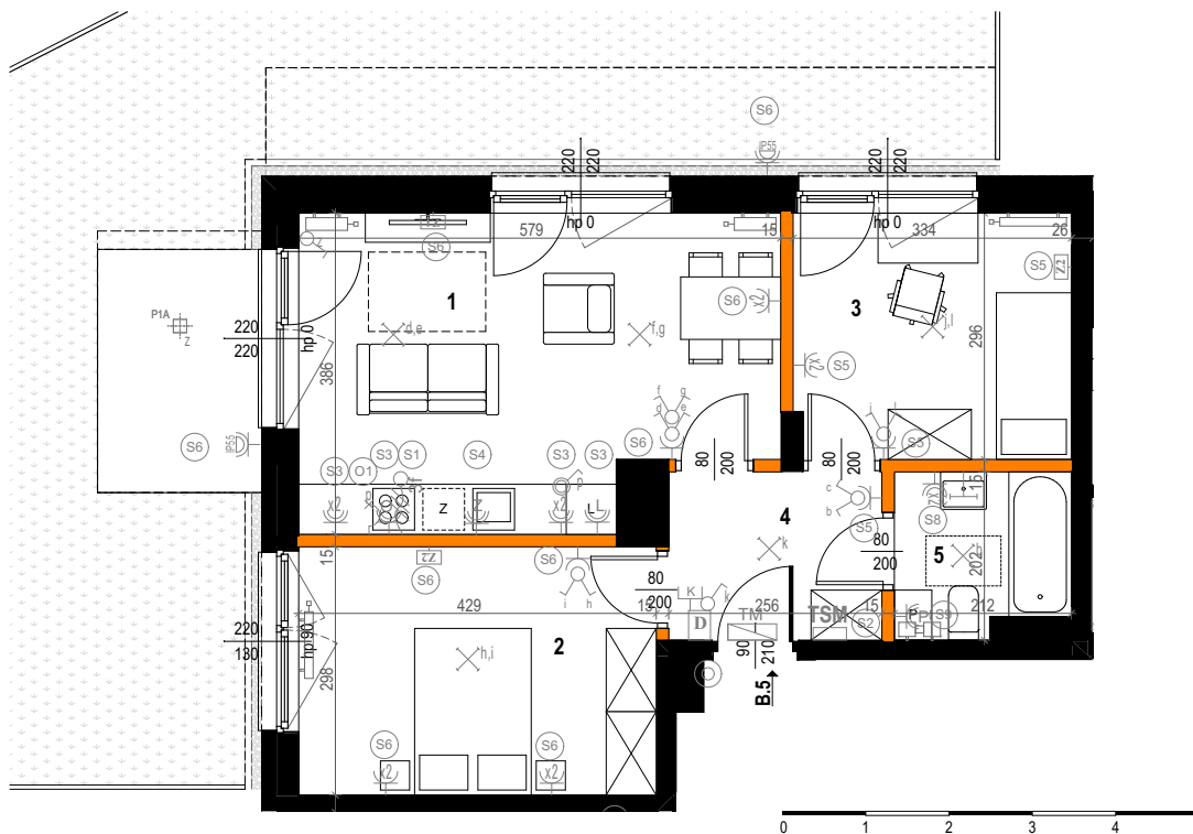
RZUT Z PRZEDOGRÓDKAMI
